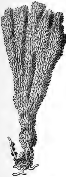
Fig. 68.— Lycopodium compactum .
